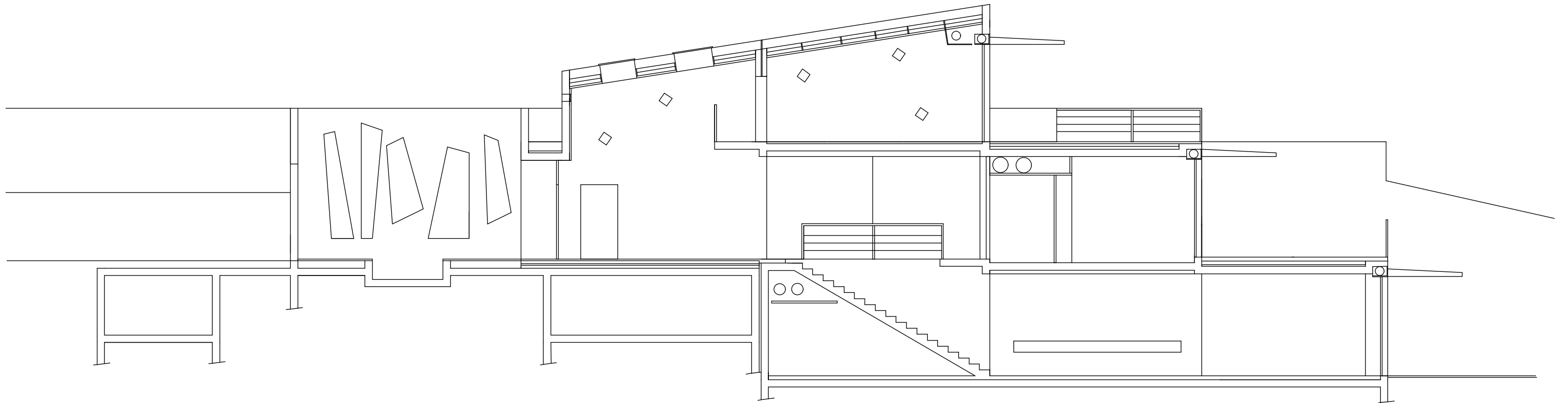
COUPE LONGITUDINALE
