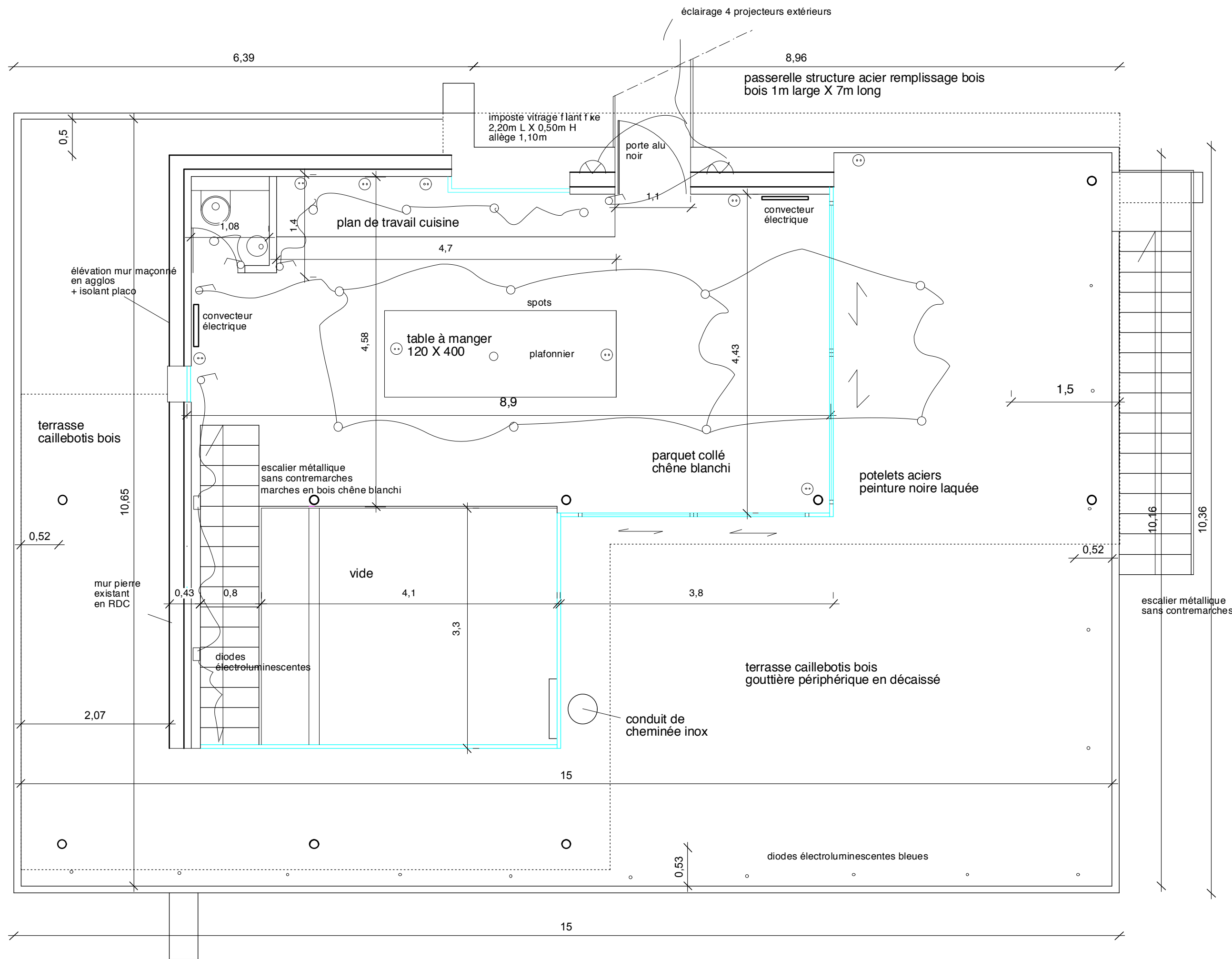
R+1 PROJETE éch 1/50°
